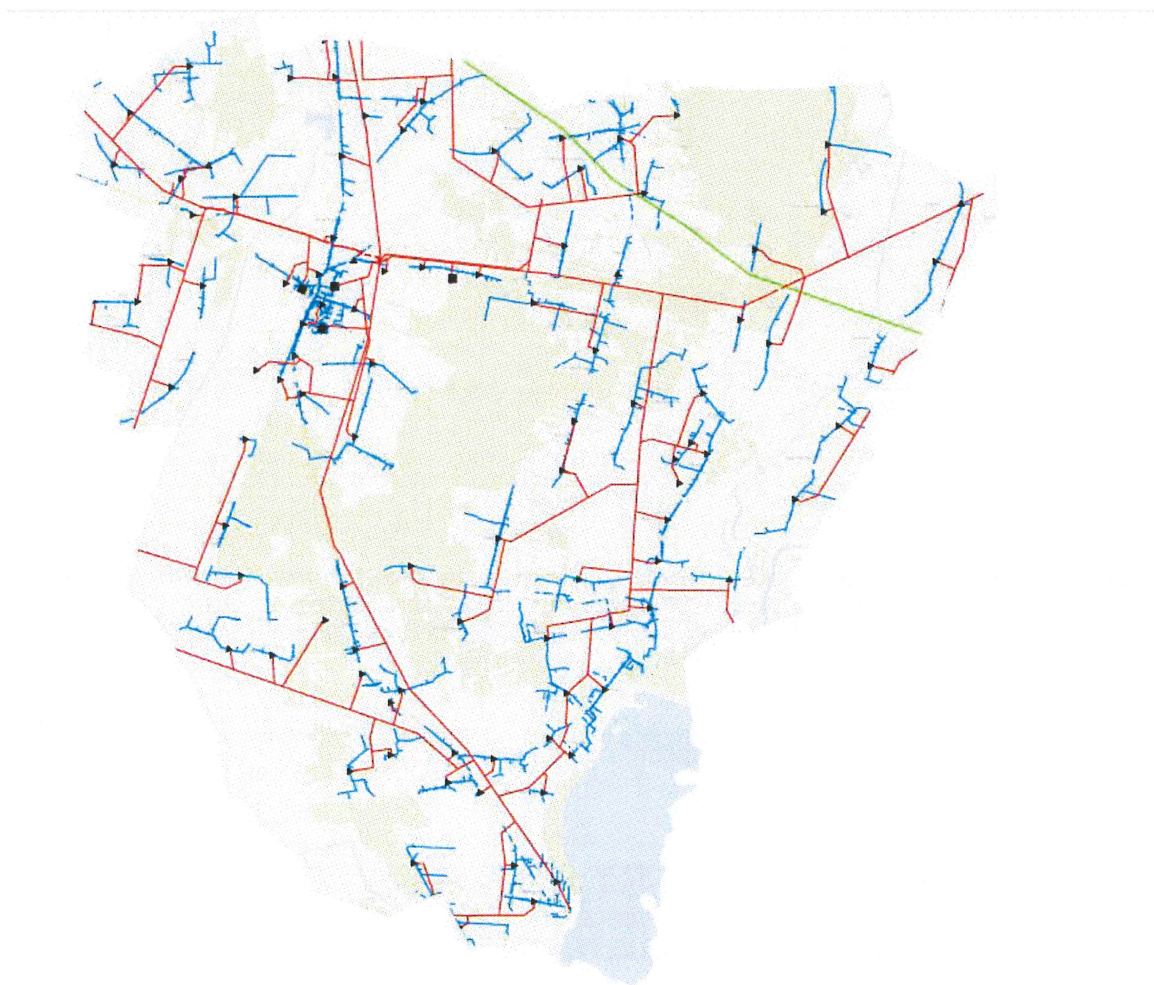
RYСУNEK 6. SCHEMAT SIECI ENERGETYCZNEJ NA TERENIE GMINY DOBRA. Źródło: ENERGA-OPERATOR S.A.
